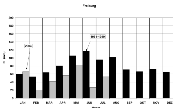
Abb. 2 und 3: Temperatur- und Niederschlagsverlauf der Wetterstation Freiburg, Jan – Juli 2003.
