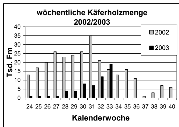
Abb. 1 zeigt die zeitliche Entwicklung des Käferholzanfalls im Gesamtwald der Forstdirektion Freiburg in den Jahren 2002 und 2003.
