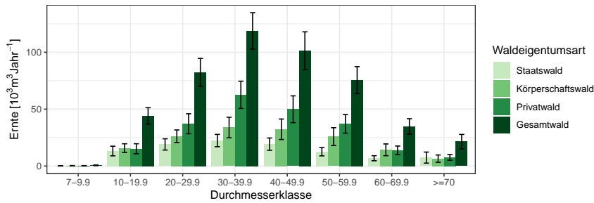
Abbildung 1.43: Nutzung [ 10^3 m^3 \text{ Jahr}^{-1} ] nach Durchmesserklasse in der Inventurperiode 2002 – 2012
