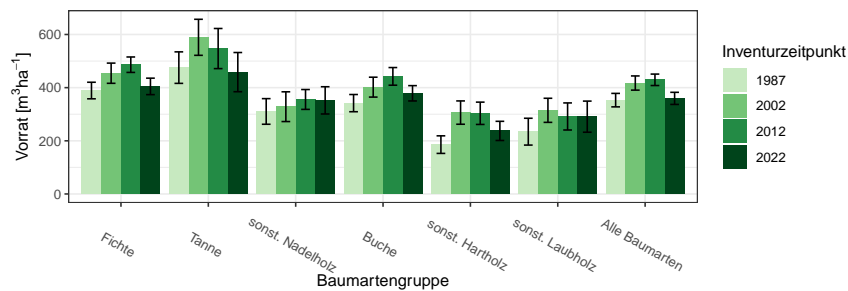
Abbildung 1.28: Vorrat [ m^3ha^{-1} ] nach Baumartengruppe und Inventurzeitpunkt im Körperschaftswald Thema: v-r-A-y-kw-kreis337
